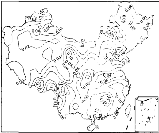
图 1 中国地表 NDVI 第 1 特征向量场
